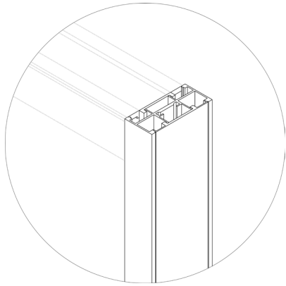
29460: P4 End Cap
