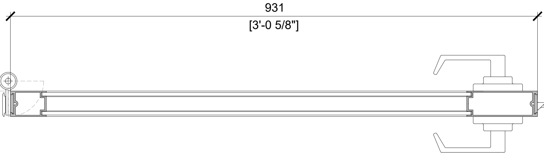
11 SWING D52 - HH45 - TERO SCALE: 1:4 (ON SIZE D - 34" X 22")
